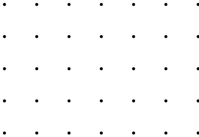
图 1.6: 正方二维布拉维格子 p 。
