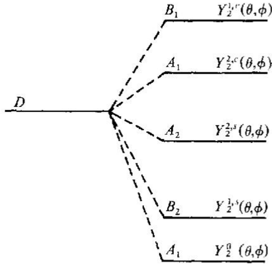
图 2.2: 原子 D 项在具有 mm2(C_{2v}) 对称性的晶体场中的示意劈裂。
