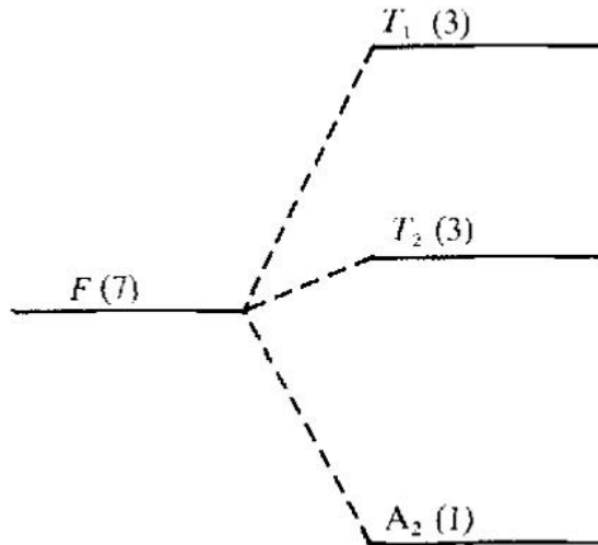
图 2.3: 原子 F 项在具有 432(O) 对称性的晶体场中的示意劈裂 (括号内给出各能级的简并度)。
